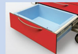
Szuflada 6 Wyposażona w wyjmowaną przegrodę Wymiary zewnętrzne, szer. x gł. x wys.: 680 x 420 x 210 mm
